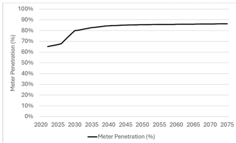
Figure 4.15: SWOX WRZ Final Plan Meter Penetration 25
